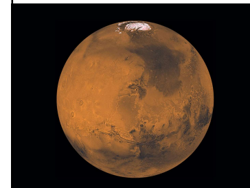
Mars
