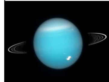
Uranus
