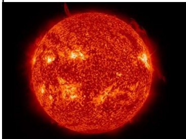
Sun
